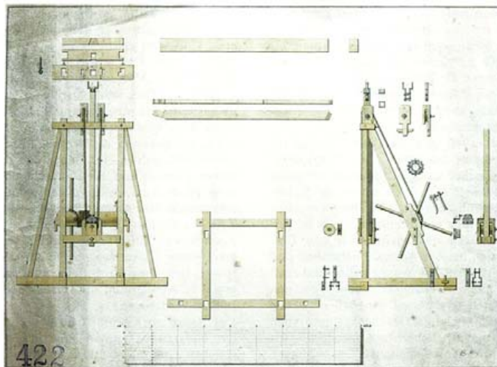
Plan eines Gerätes zum Umpflanzen besonders großer und schwerer Pflanzen
