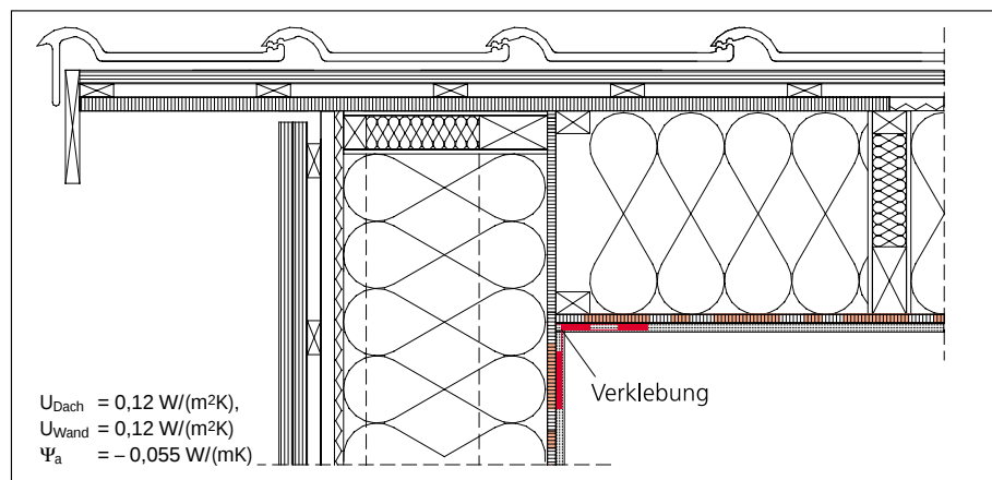
Abbildung 8 Ortgang. Die Innenbeplankung aus Holzwerkstoff-Platten bildet die luftdichte Ebene. An den Stößen und Kanten werden die Platten mit Folienstreifen oder luftdichter Baupappe flächig verklebt.
