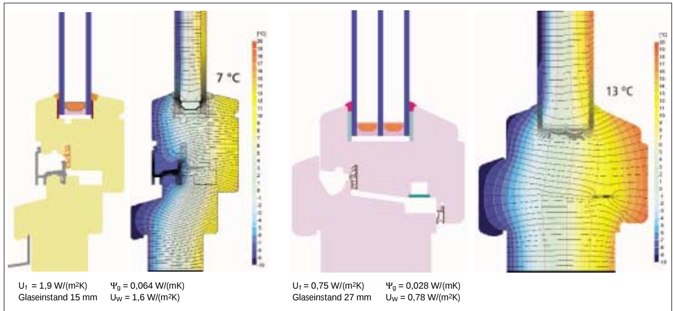
Abbildung 19 Standard-Fensterrahmen (IV68) aus Nadelholz im Vergleich zu einem wärmegeprägten Fensterrahmen, jeweils mit Isothermenbild. Beim gedämmten Rahmen sind Glaseinstand (20...30 mm) und Bautiefe (hier 120 mm) vergrößert, ein thermisch getrennter Randverbund wird verwendet. Stellvertretend für viele mögliche Konstruktionen [ 28 ] ist im Bild ein fiktives homogenes Material ( \lambda = 0,085 \text{ W/(mK)} ) eingezeichnet. Man beachte besonders die Oberflächentemperaturen am Glasrand innen: 7 °C im Auslegungsfall führen beim ungedämmten Standard-Fensterrahmen mit Alu-Randverbund regelmäßig zu Tauwasserbildung. Beim gedämmten Rahmen ist dies nicht der Fall.
