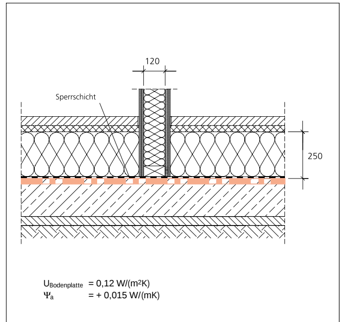
Abbildung 11 Innenliegende Dämmung. Die luftdichte Schicht ist wieder die Betonplatte. Über der Betonplatte muß eine Sperre gegen aufsteigende Feuchte vorgesehen werden. Als raumseitige Feuchte-Sperre dient die Folie unter dem Estrich.
