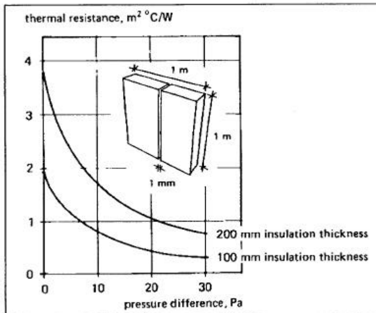
Abbildung 2: Luftströmungen durch undichte Hüllflächen
