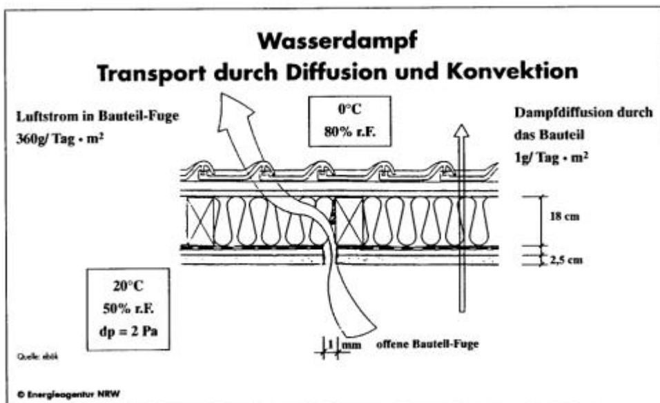
Abbildung 1: Wasserdampftransport durch einen Dachaufbau
