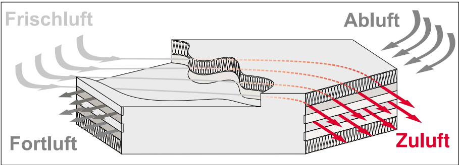
Abbildung 23 Der Wärmeübertrager, Herzstück der kontrollierten Wohnungslüftung mit Wärmerückgewinnung. Zuluft- und Abluftkanäle sind vollständig voneinander getrennt.
